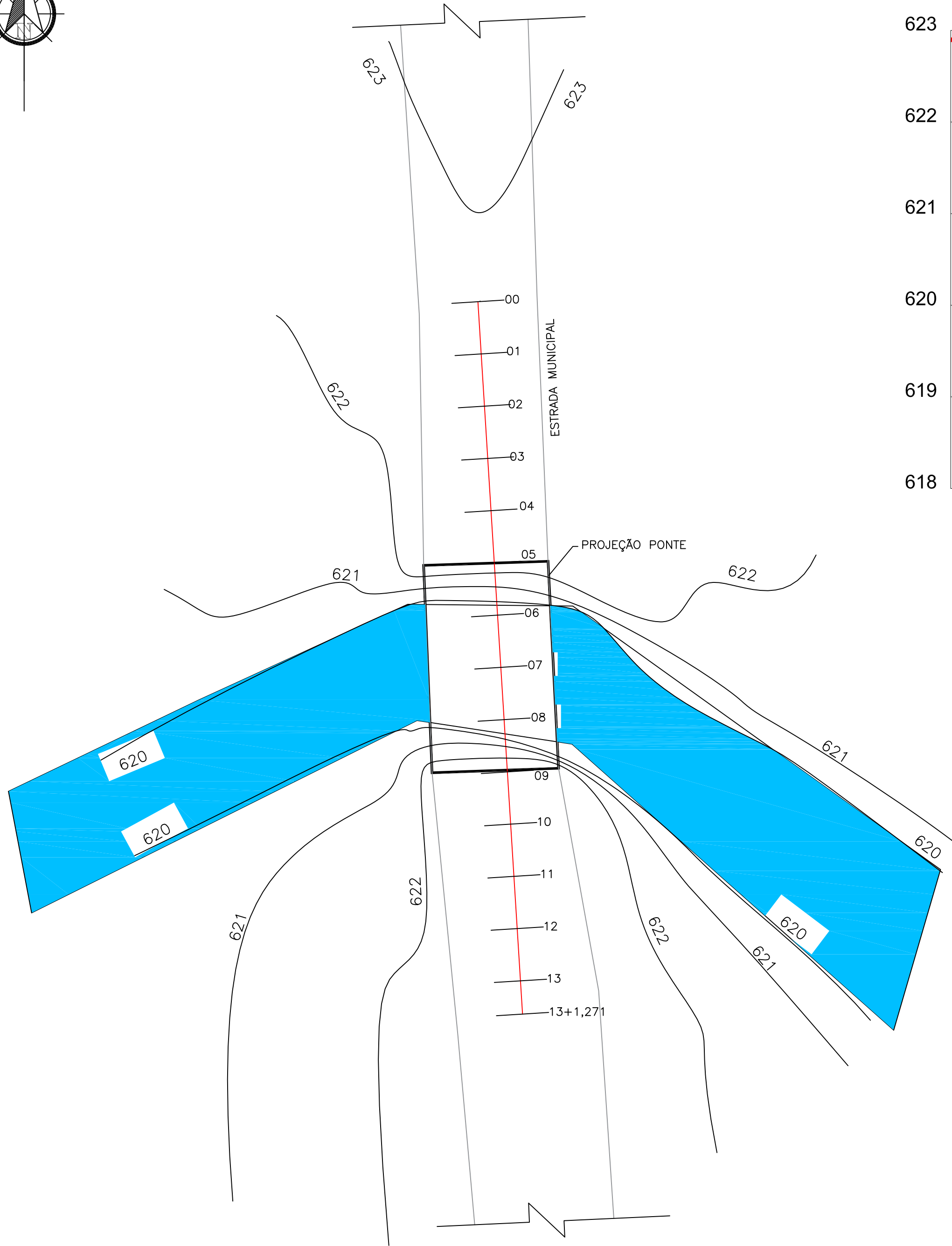
PROJETO TOPOGRÁFICO esc 1/50
