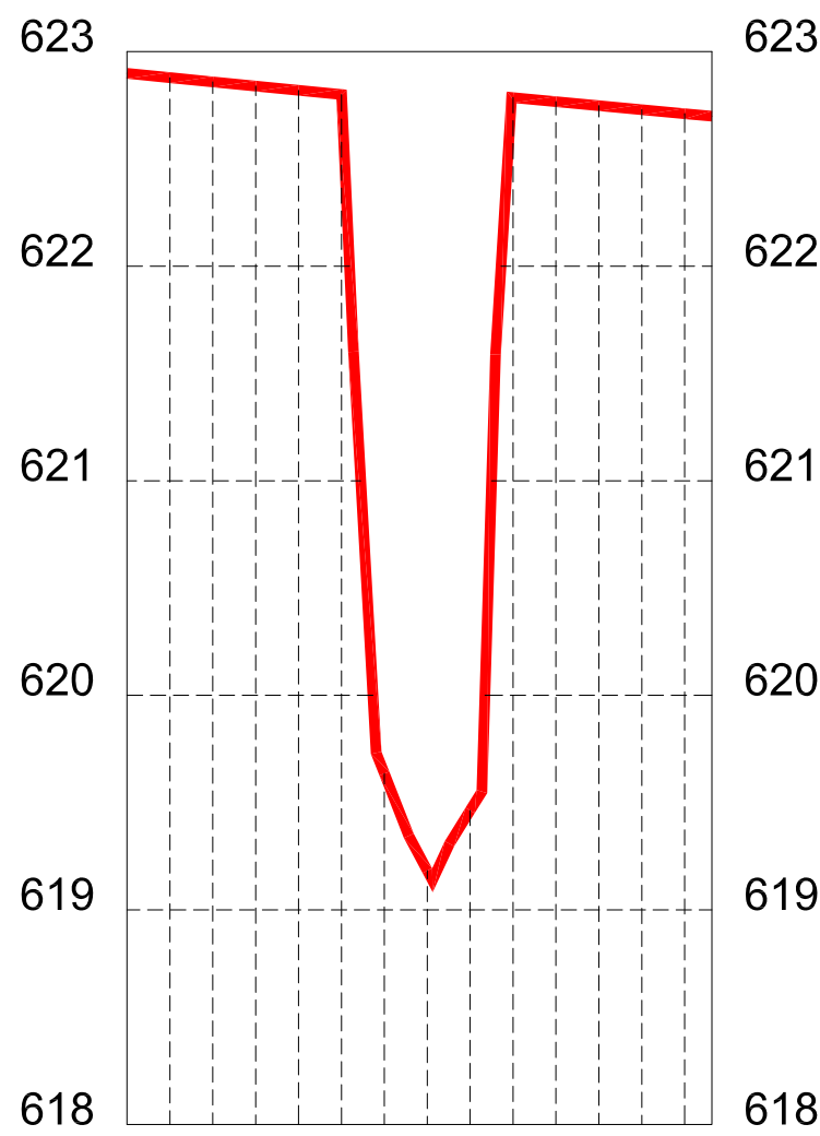
PERFIL DO TERRENO esc 1/50
