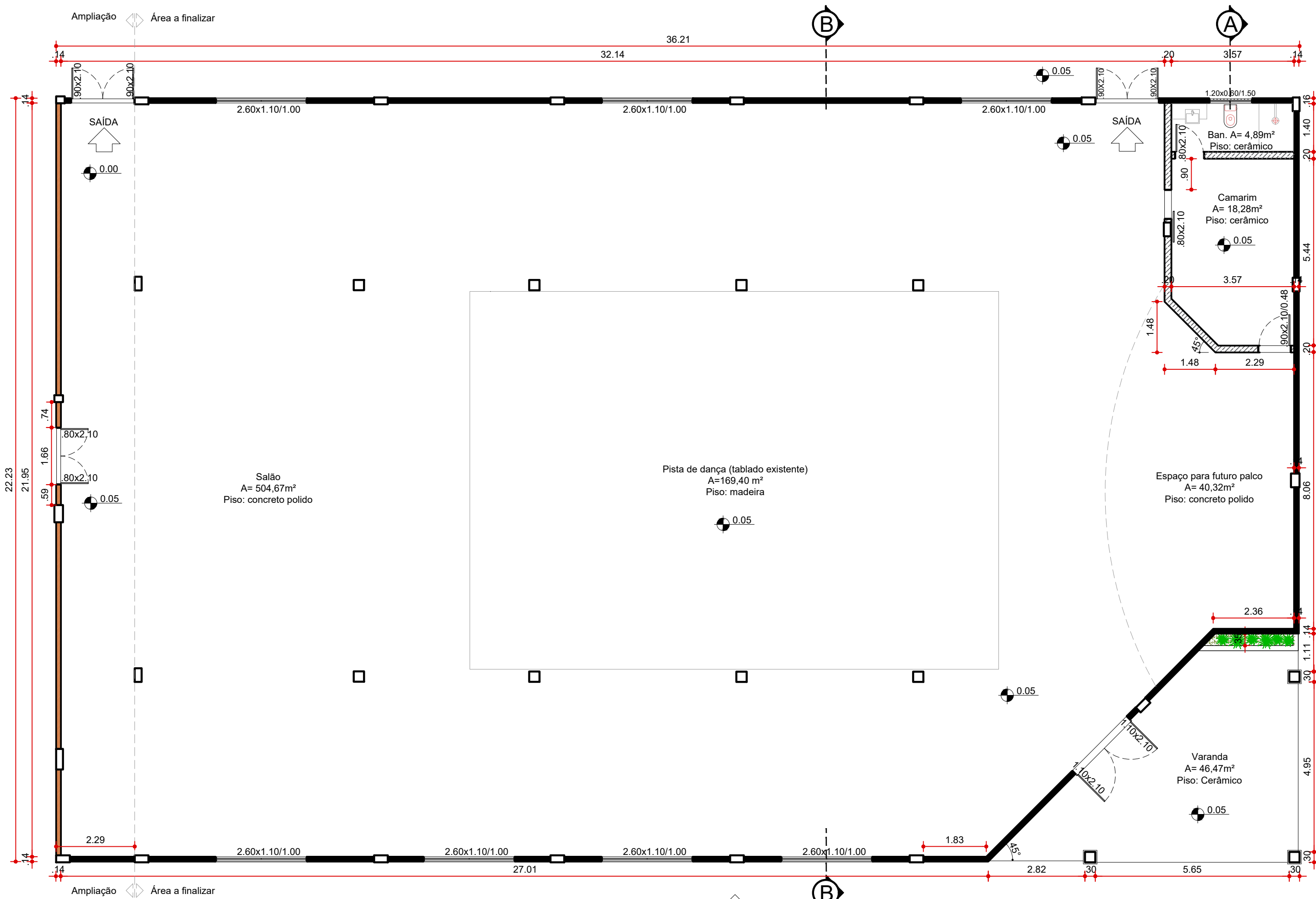
01. PLANTA BAIXA esc: 1/100
