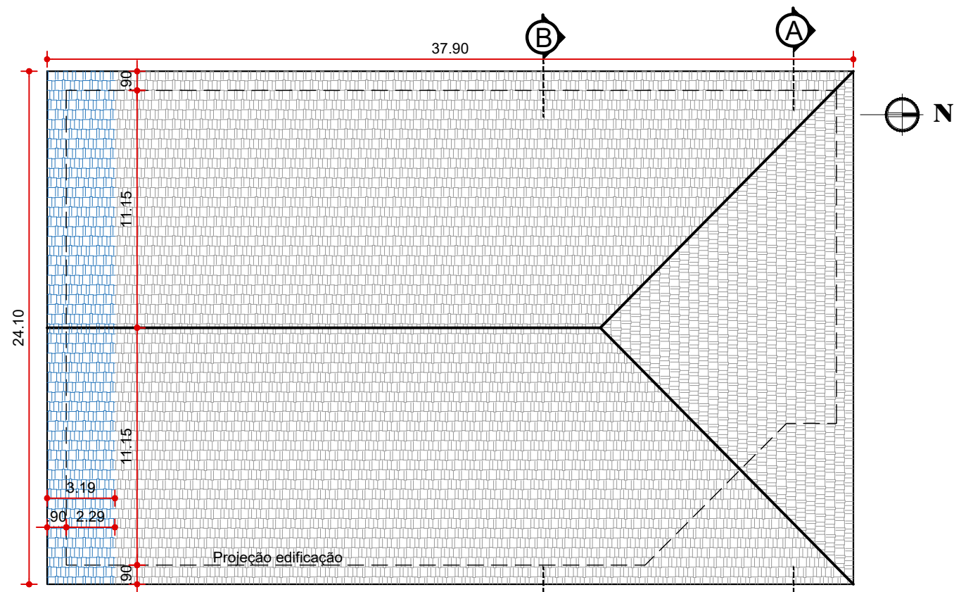
02. PLANTA DE COBERTURA esc: 1/250
