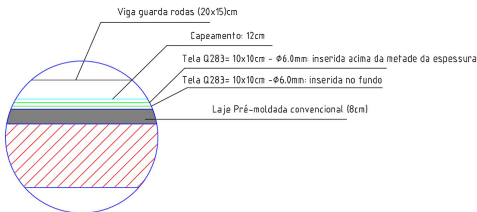
DETALHE- Capeamento
