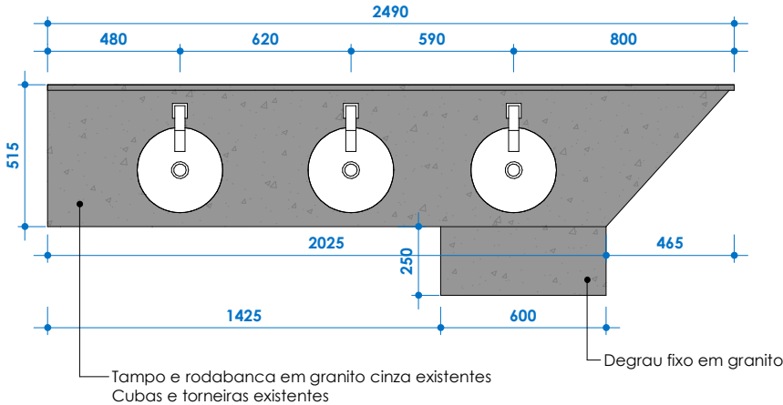
VISTA SUPERIOR ESC: 1 : 25
