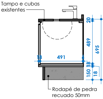
CORTE TRANVERSAL ESC: 1 : 25
