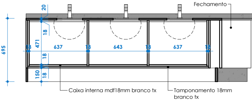
VISTA FRONTAL ABERTA ESC: 1 : 25
