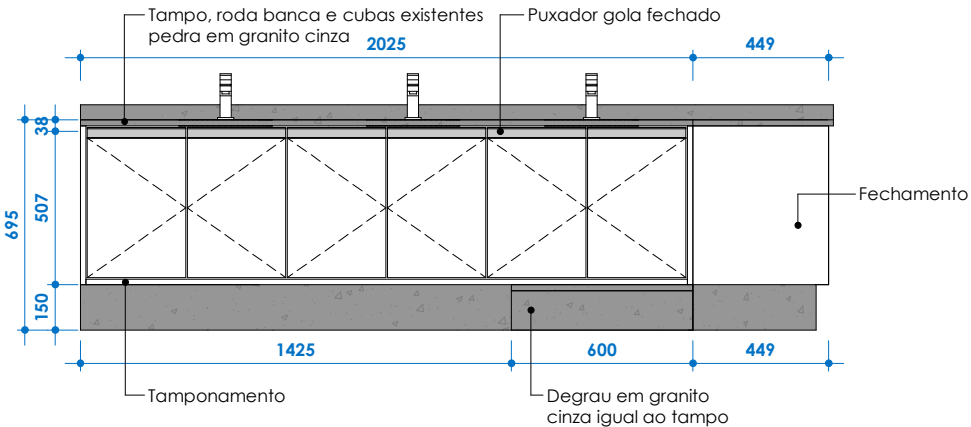
VISTA FRONTAL ESC: 1 : 25
