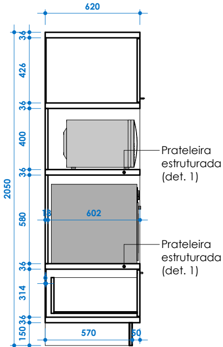
CORTE TRANVERSAL ESC: 1 : 25
