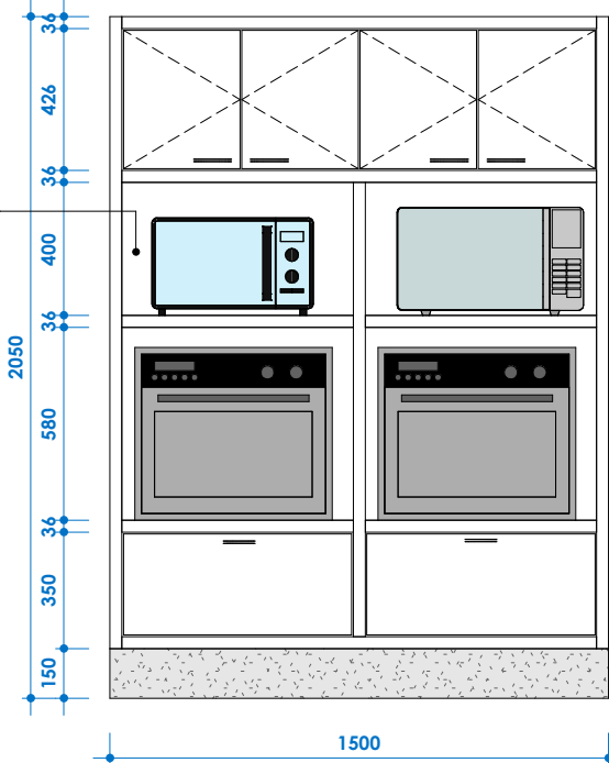
VISTA FRONTAL ESC: 1 : 25
