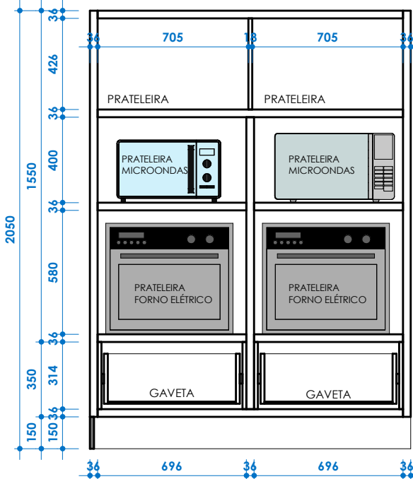
VISTA FRONTAL ABERTA ESC: 1 : 25
