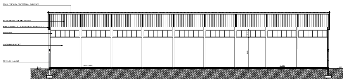
05. CORTE BB' esc: 1/125
