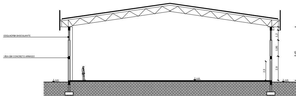
03. CORTE AA' esc: 1/125
