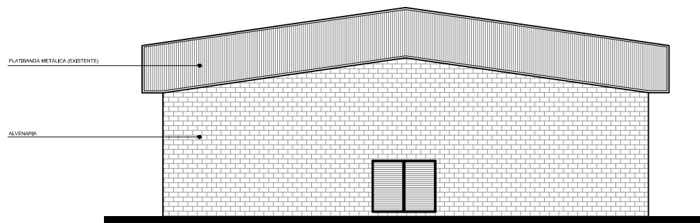
04. FACHADA SUL esc: 1/125
