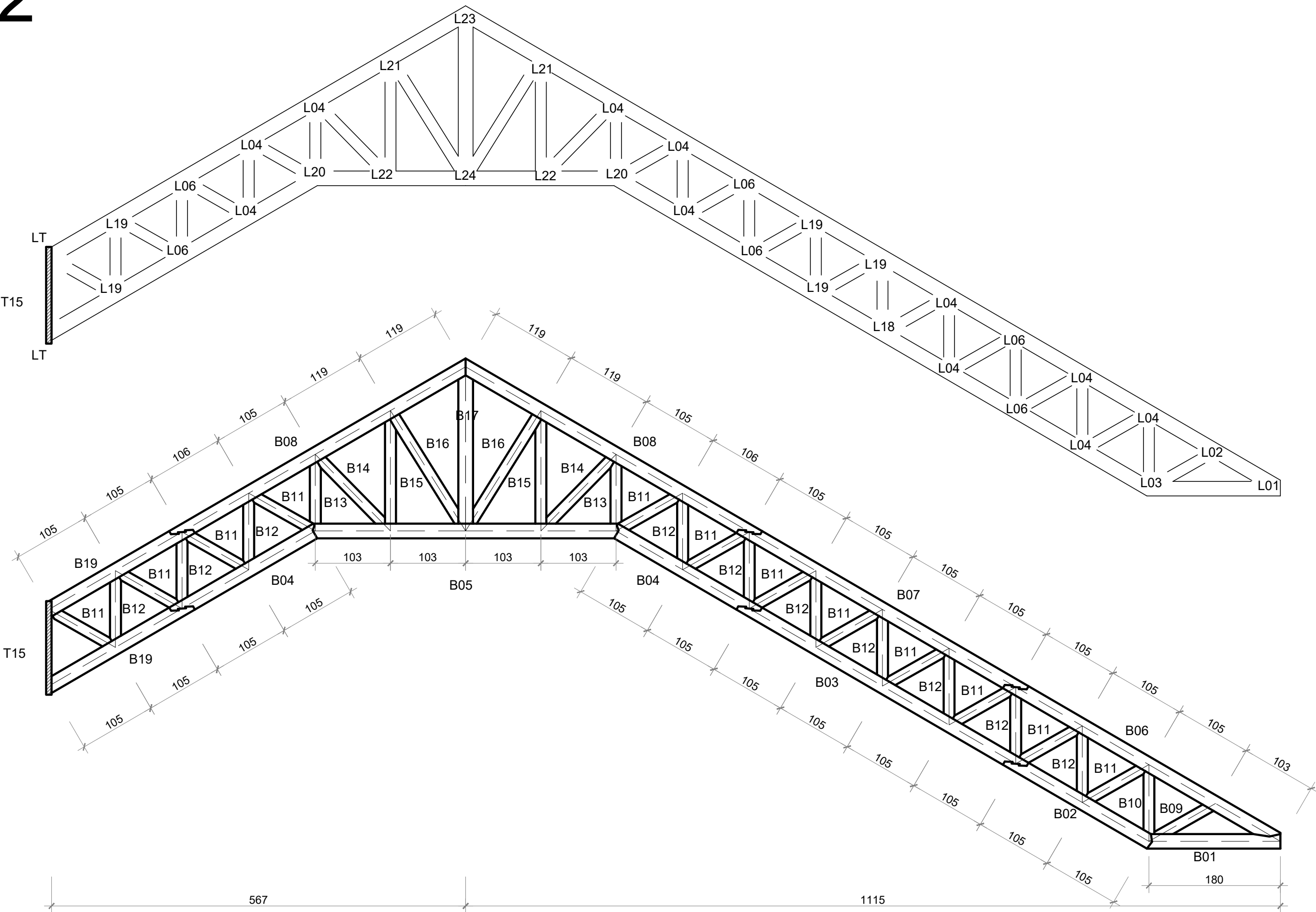
1 Treliça escala 1:50
