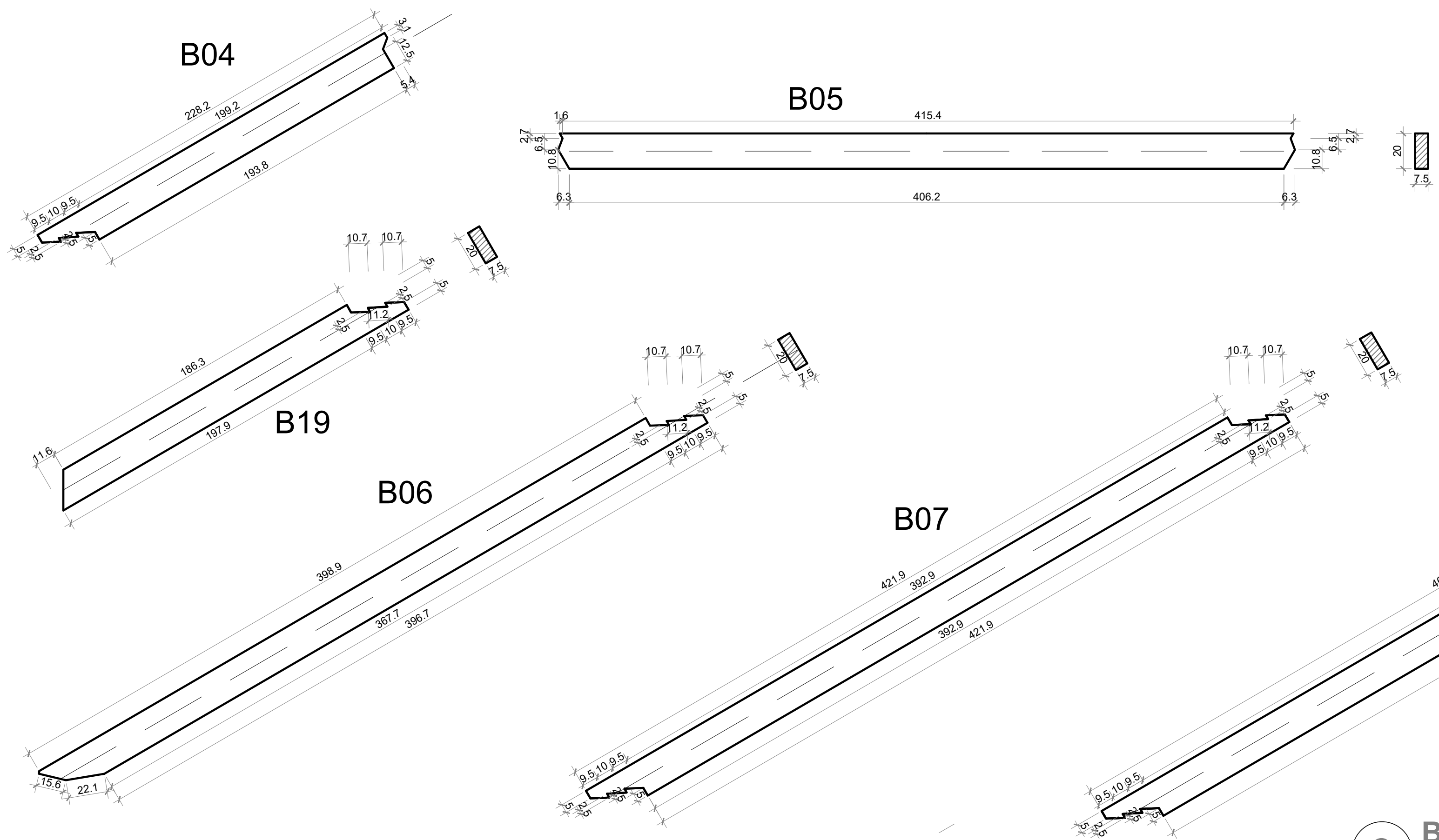
1 Treliça escala 1:50
