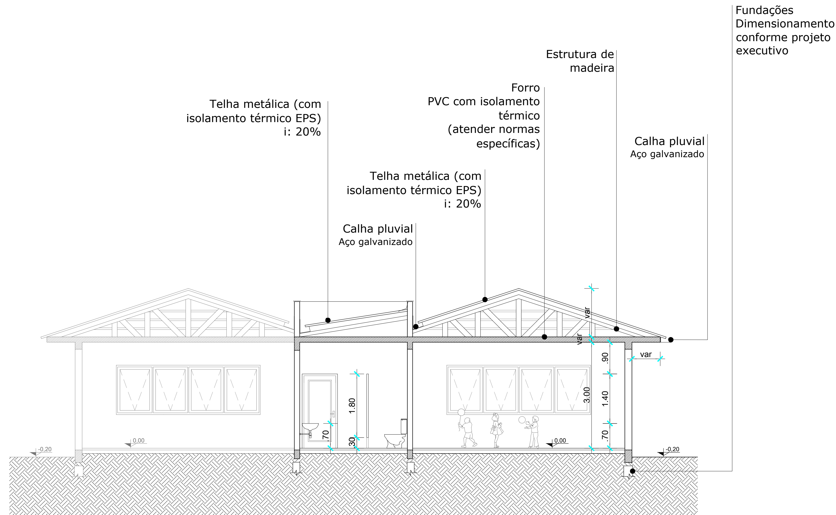
07. CORTE BB' esc: 1/75
