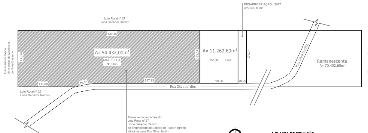
01. PLANTA DE SITUAÇÃO esc: 1/2000
