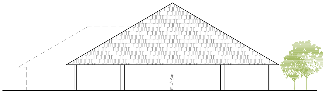
05 | FACHADA — esc: 1/75
