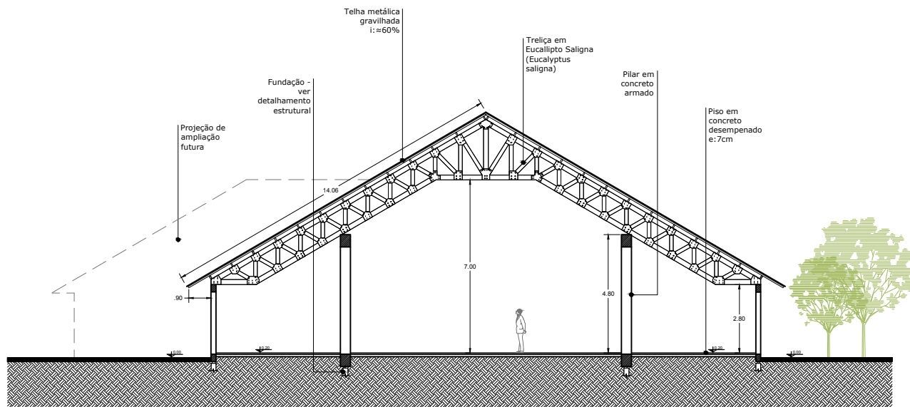
04 | CORTE AA' — esc: 1/75
