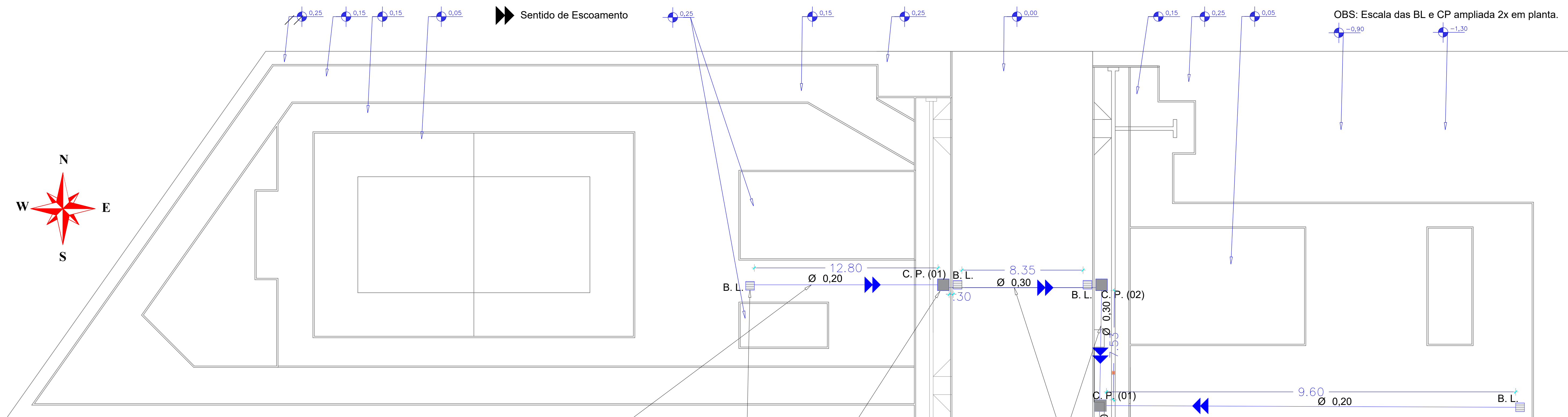
PLANTA DE DRENAGEM Escala 1/ 140
