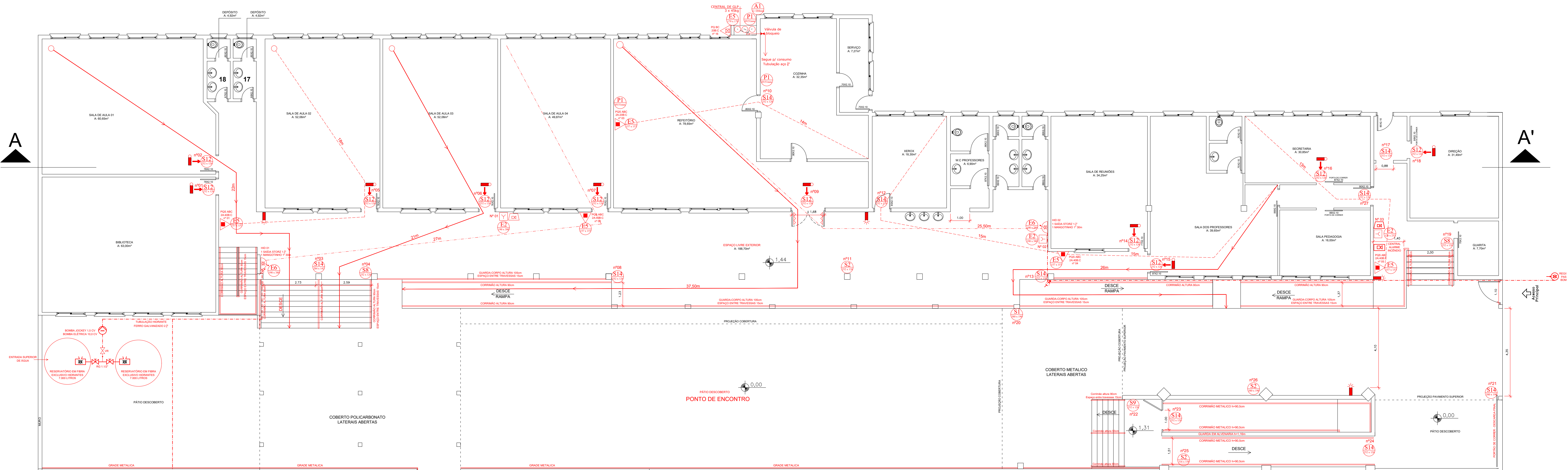
PLANTA BAIXA TERREO A: 1031,68m² esc. 1/100
