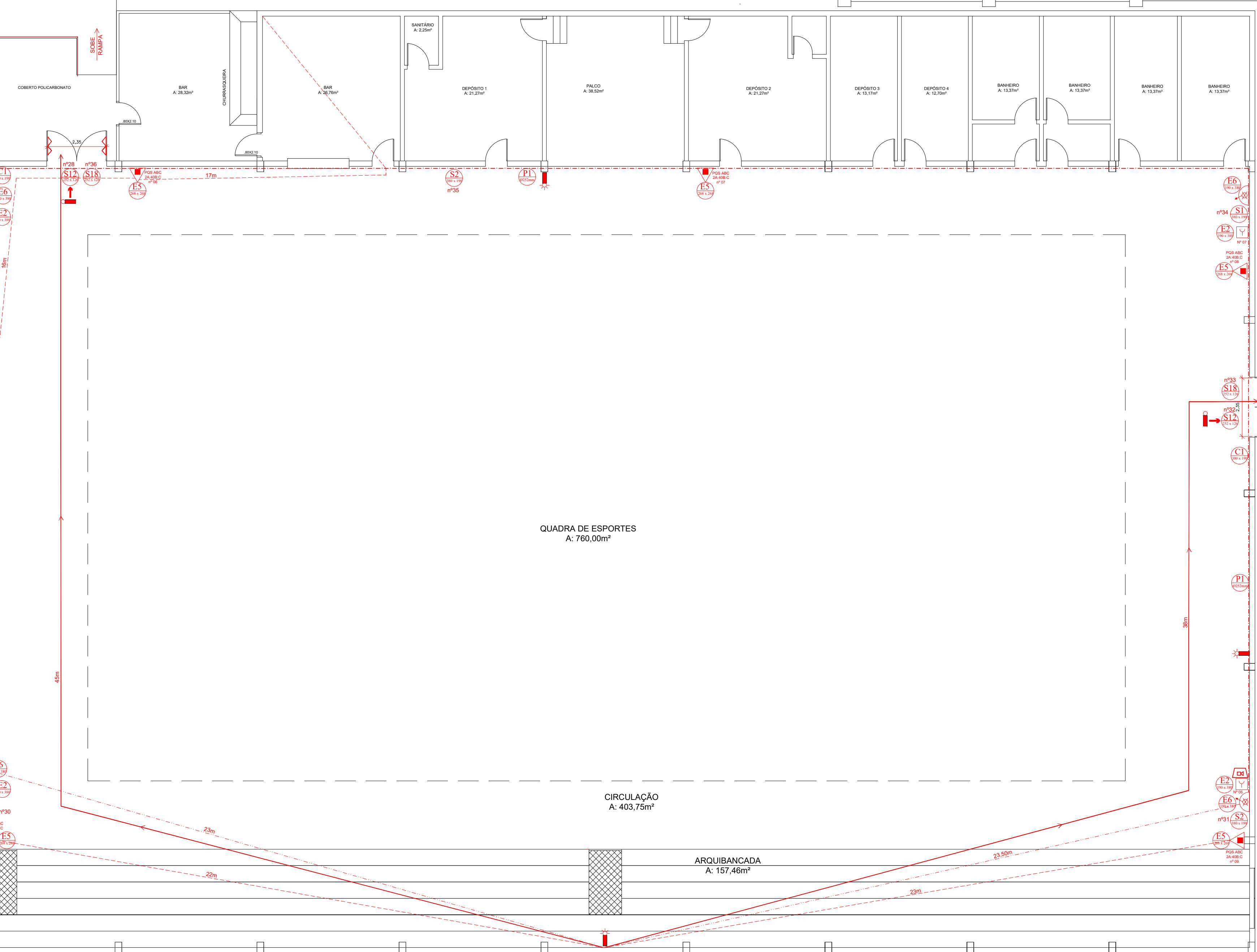
PLANTA BAIXA GINÁSIO TÉRREO A: 1.590,90m² esc. 1/100
