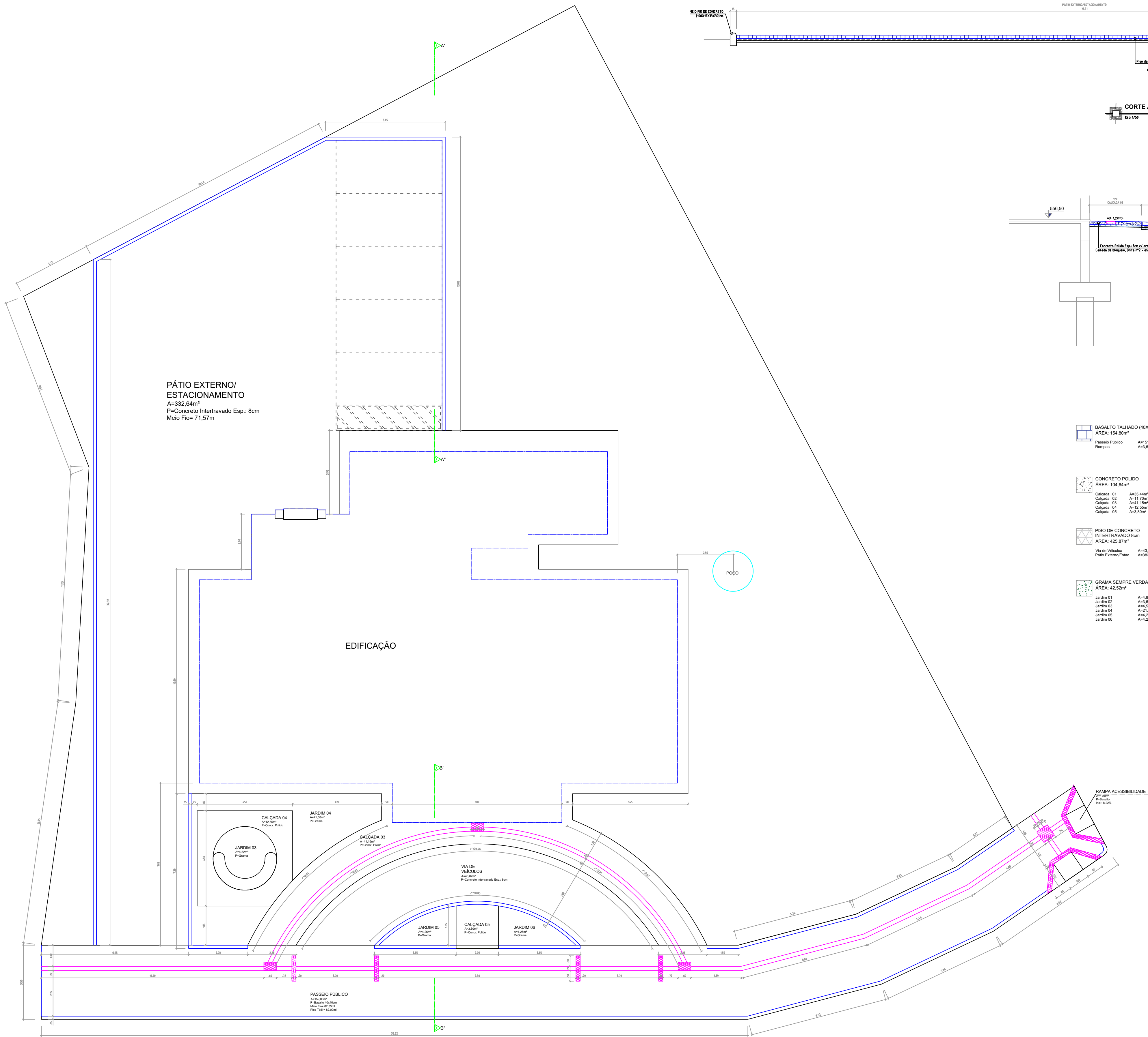
Projeto Geométrico PAVIMENTAÇÃO/ACESSIBILIDADE Esc: 1/100
