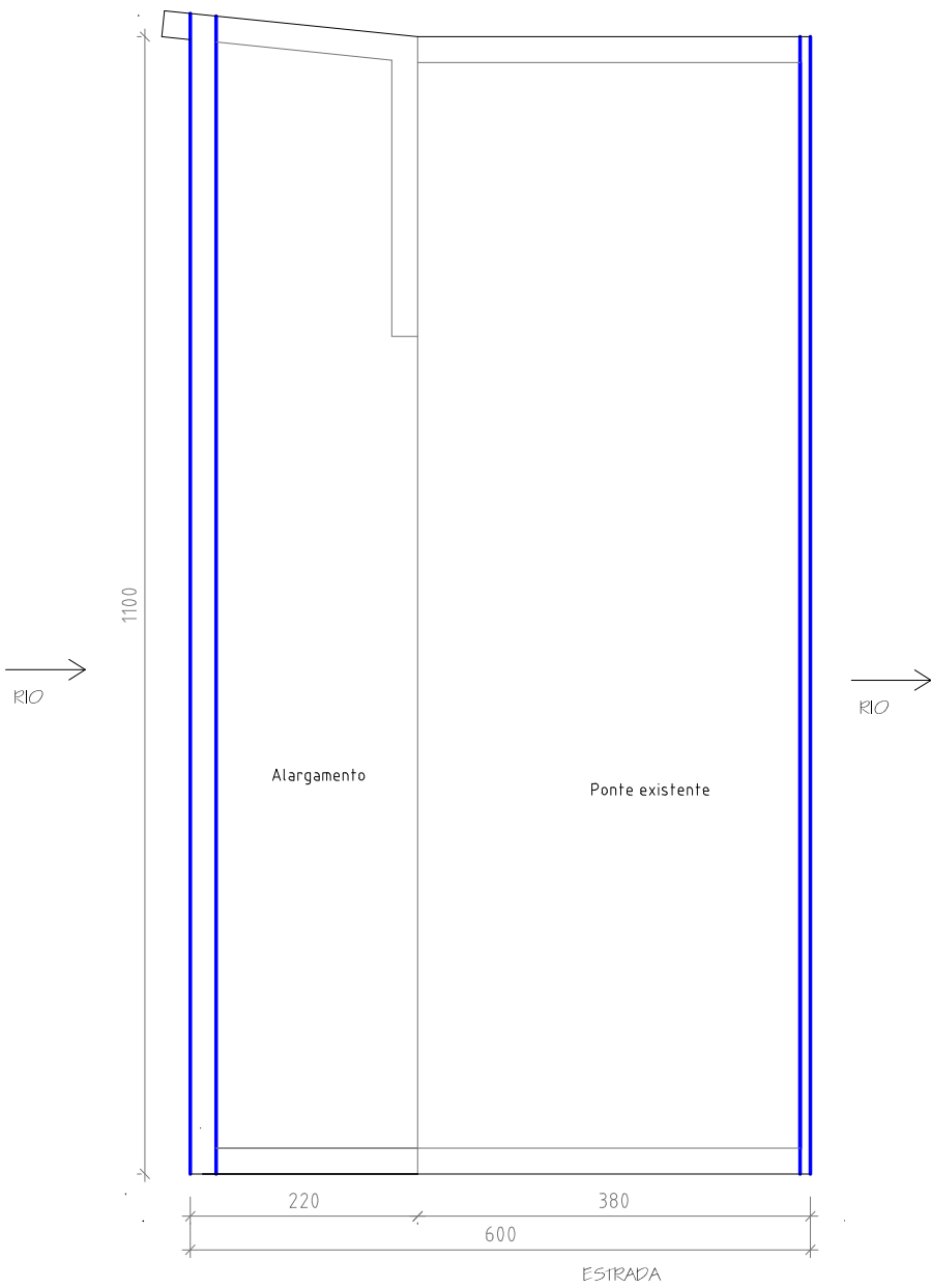
PLANTA BAIXA Ponte São Pedro- Ponte 04 Área= 24,20m² Esc 1:75
