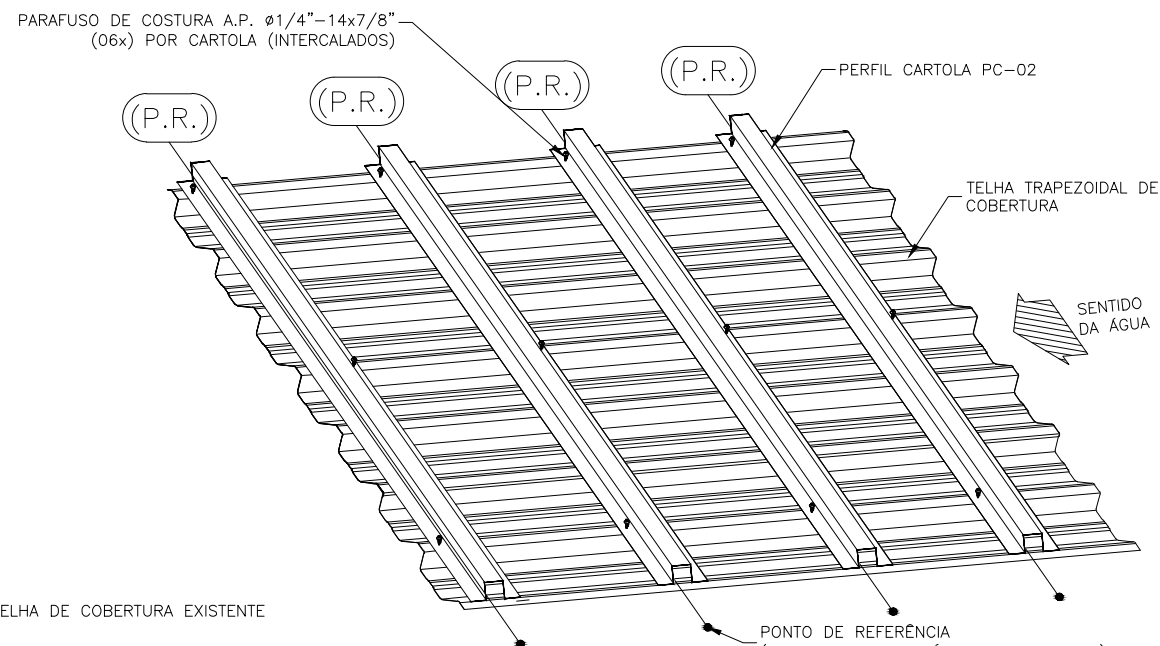
2*) FIXAÇÃO DO CARTOLA PC-02
