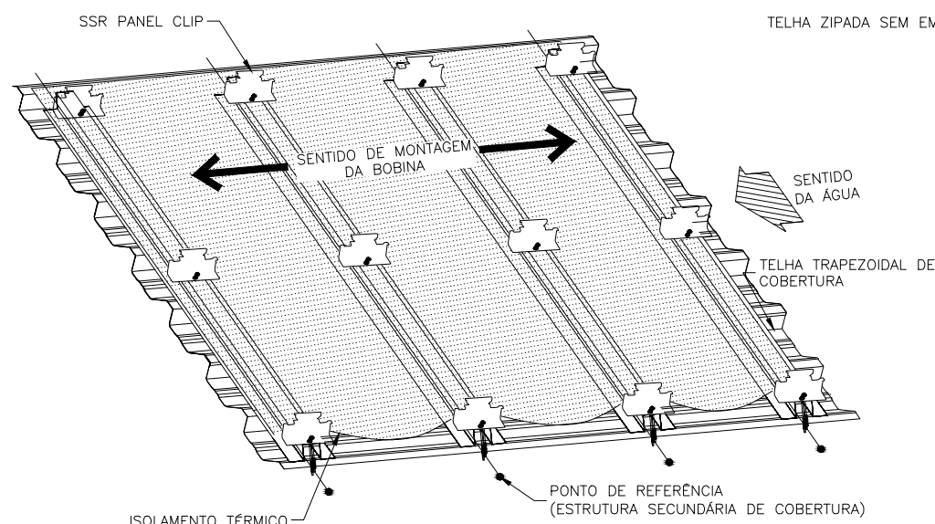
3*) MONTAGEM DO ISOLAMENTO TÉRMICO E FIX. DOS CLIPS
