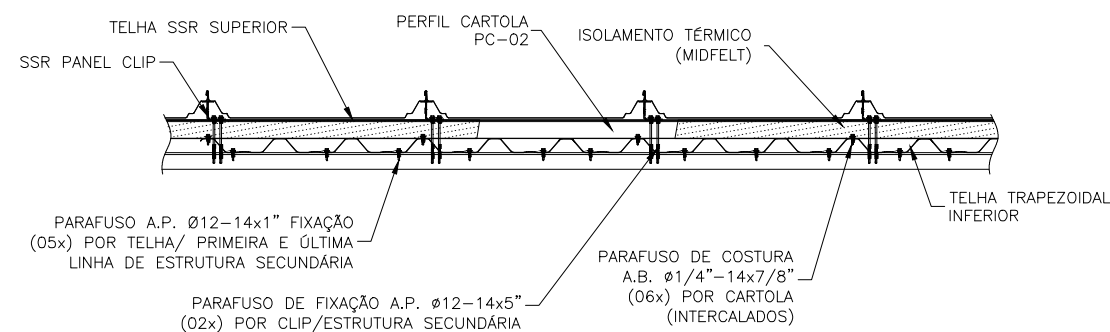
DETALHE TÍPICO DE FIXAÇÃO DA TELHA SANDUÍCHE NA ESTRUTURA SECUNDÁRIA NO TRANSPASSE TRANSVERSAL E NAS EXTREMIDADES
