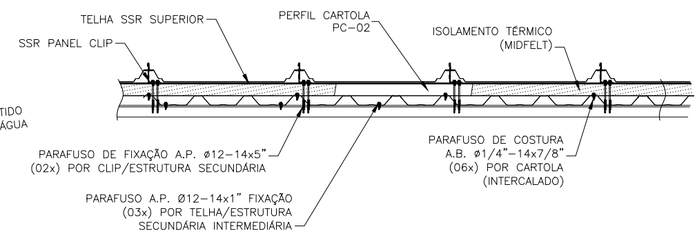
DETALHE TÍPICO DE FIXAÇÃO DA TELHA SANDUÍCHE NA ESTRUTURA SECUNDÁRIA INTERMEDIÁRIA
