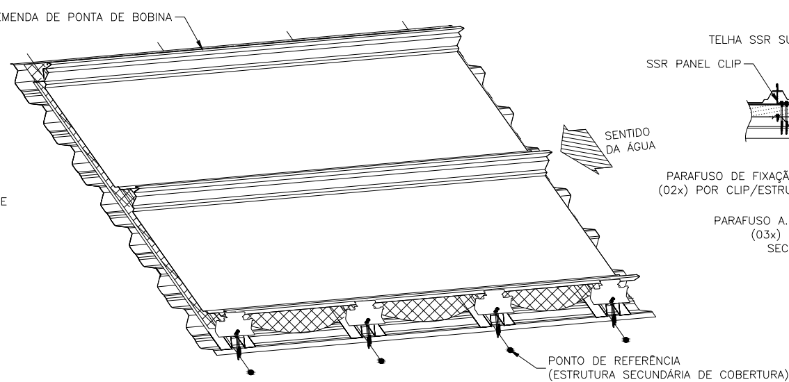
4*) MONTAGEM DA TELHA SSR SISTEMA SANDUICHE DE COBERTURA
