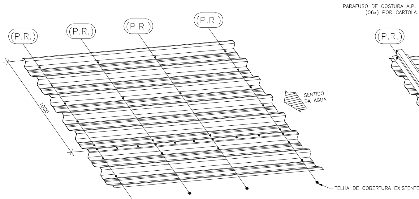
1*) FIXAÇÃO DA TELHA PANEL RIB III INFERIOR (EXISTENTE)
