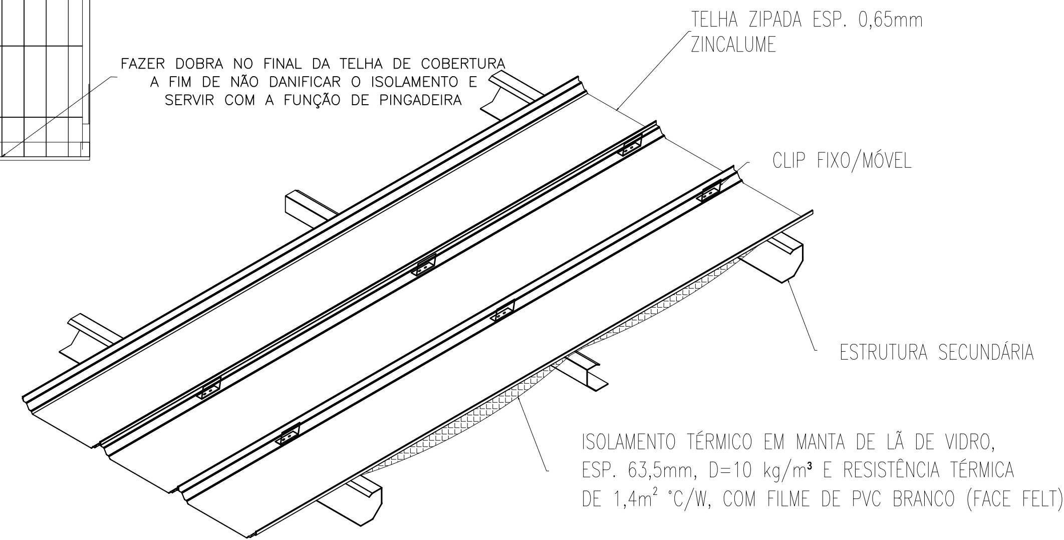
DETALHE DA TELHA DE COBERTURA ESC.:1/ 20
