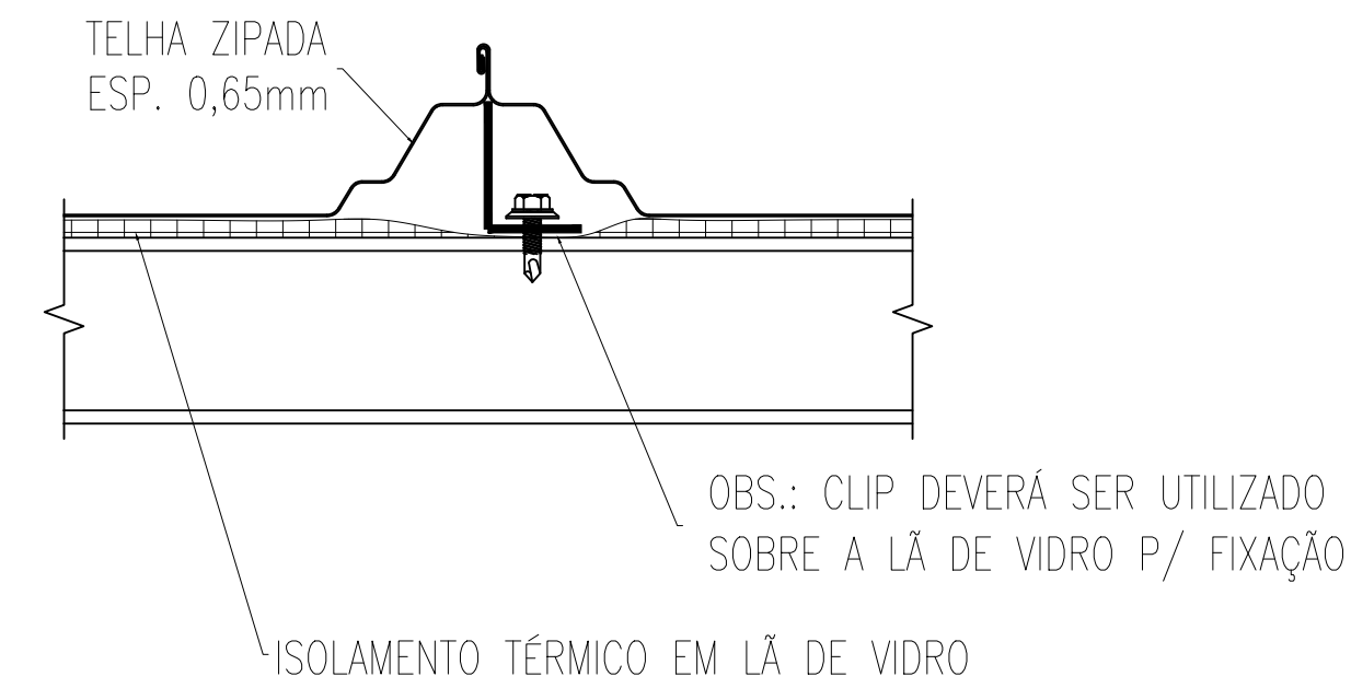
DETALHE DE FIX. DO CLIP ESC.:1/ 5
