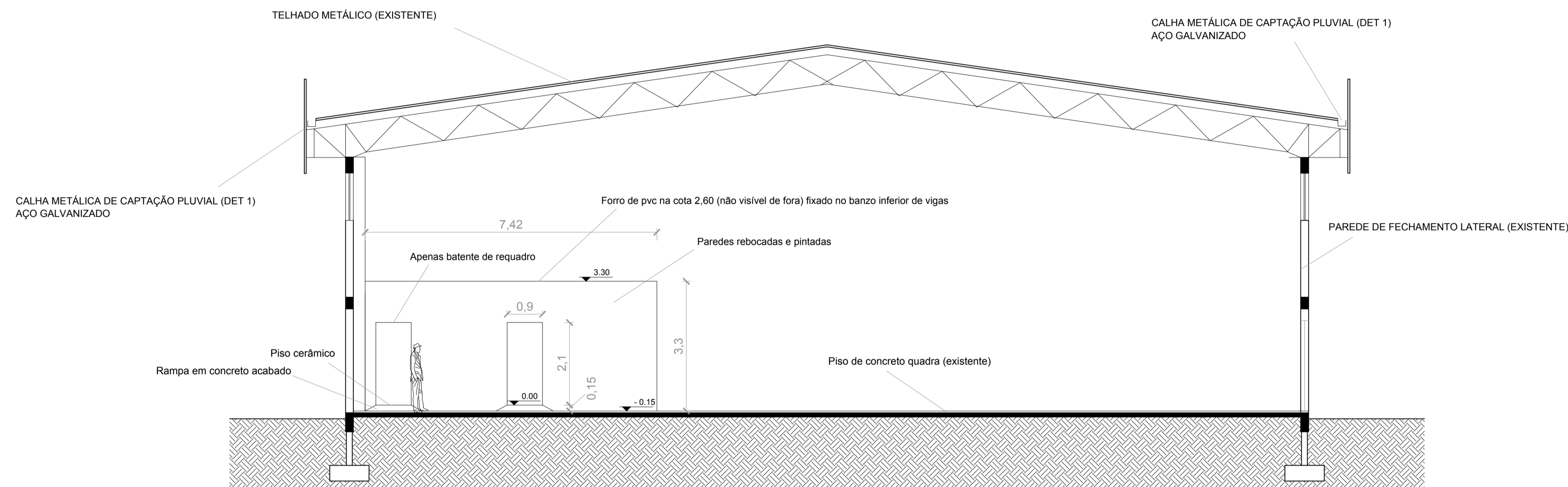
05. CORTE AA' esc: 1/125
